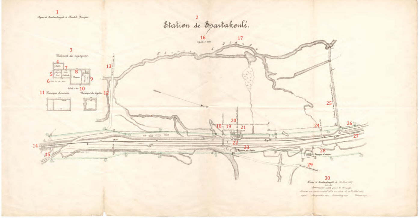
Tren 1: İstanbul-Kuleliburgaz yolu Ispartakule İstasyonu planı (Fr.) BOA, PLK.p, 6157
